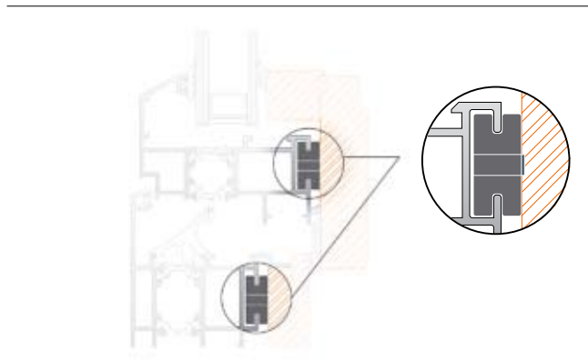
Ειδικός σύνδεσμος μεταξύ αλουμινίου και ξύλου, που επιτρέπει την αυτόνομη προσαρμογή του κάθε υλικού στις θερμοκρασιακές μεταβολές
